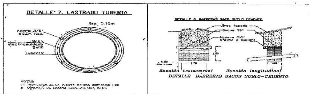
Imagen No. 13: Esquema de obras de geotecnia y bajado de tubería. Fuente: SOLICITUD DE PERMISO DE OCUPACIÓN DE CAUCE, Caño Vida Tranquila, 2021.
