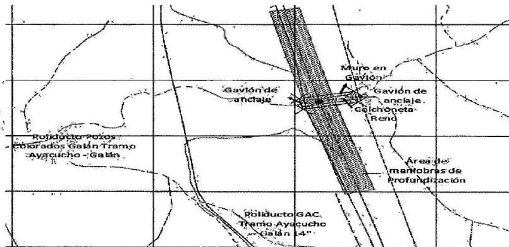
Imagen No. 12: Obras de geotecnia y bajado de tubería Combustoleoducto Galán - Ayacucho 18" PK 142+500 (CGA - 18)". Fuente: SOLICITUD DE PERMISO DE OCUPACIÓN DE CAUCE, Quebrada NN 2021.
