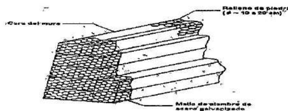
Imagen No. 11: Componentes del Gavión. Fuente: Universidad Católica de Colombia 9 .
