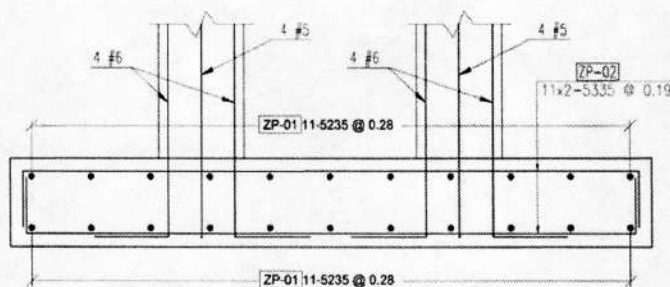
Ilustración 7. Refuerzo de zapatas de cimentación del Puenteducto.
