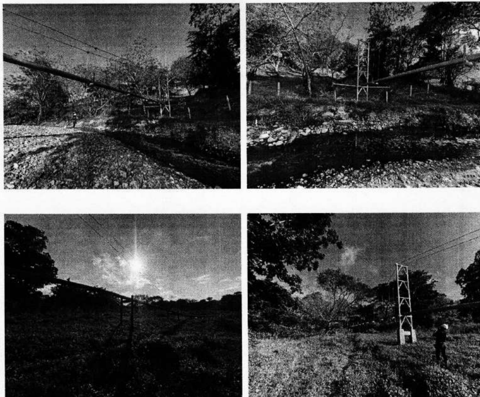
Ilustración 2. Estado ACTUAL del Puenteducto construido como obras de defensa sin permiso, en el cruce del Oleoducto Ayacucho – Galán 8” en PK 155+510 con el Arroyo Quebradita. Fuente: Propia.
