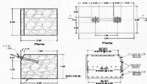
Ilustración 9. Bloque de anclaje margen derecho y detalle de reforzamiento.
