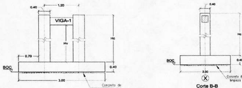
Ilustración 6. Zapatas de cimentación del Puenteducto.
