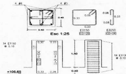
Ilustración 8. Detalle de columnas y su acero de refuerzo, construidas sobre las zapatas de cimentación.
