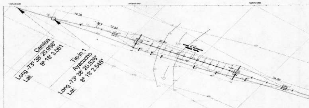
Ilustración 5. Vista en planta del Puenteducto construido sobre el Arroyo Quebradita.
