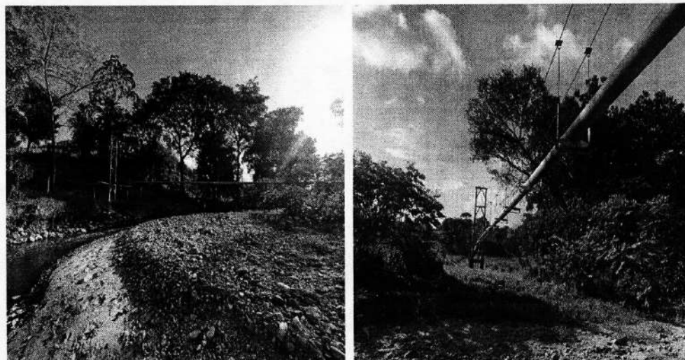
Ilustración 1. Estado del ANTES del Puenteducto en el PK 155+510 Oleoducto Ayacucho – Galán 8", que cruza el Arroyo Quebradita 1 .
