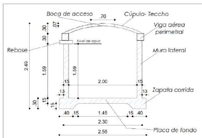
Imagen 15. Esquema de diseño del sistema de abastecimiento de aguas lluvias
