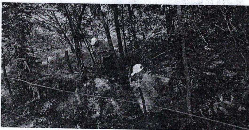
Imagen 3. Aforo de caudal por el método del flotador en el canal del predio La Voluntad.
