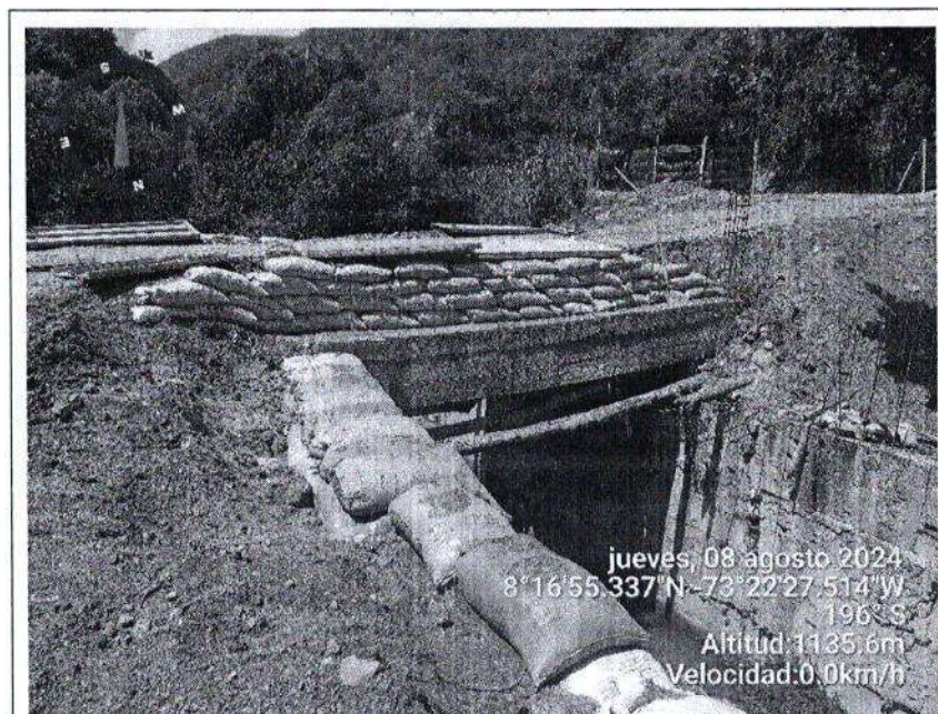
Imagen 2. Vista lateral del puente y muros en concreto e instalación de costales rellenos de material. Fuente: Autores.
