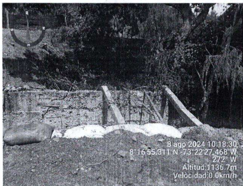
Imagen 3. Vista frontal en la construcción de muro de contención en concreto.
