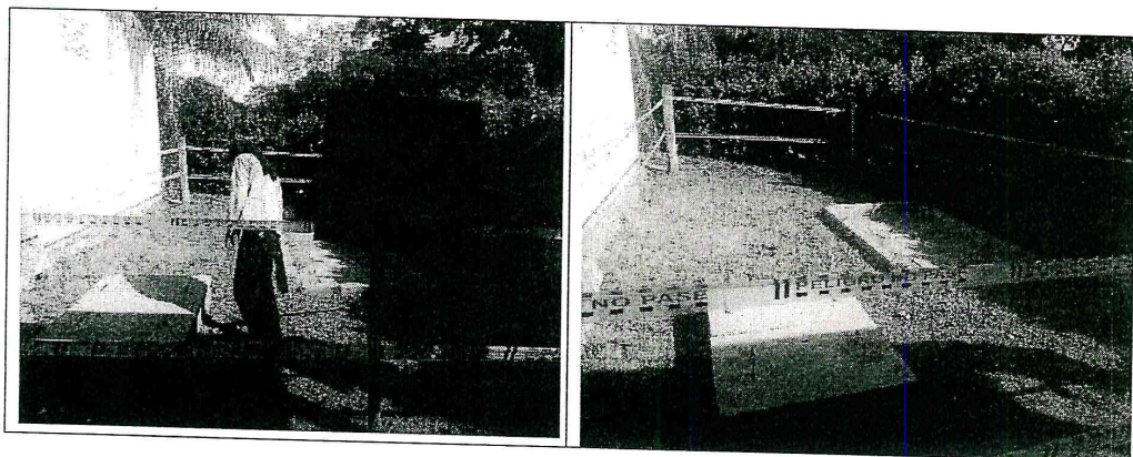
Ilustración 8. Trampa de grasa y pozo séptico área cocina
