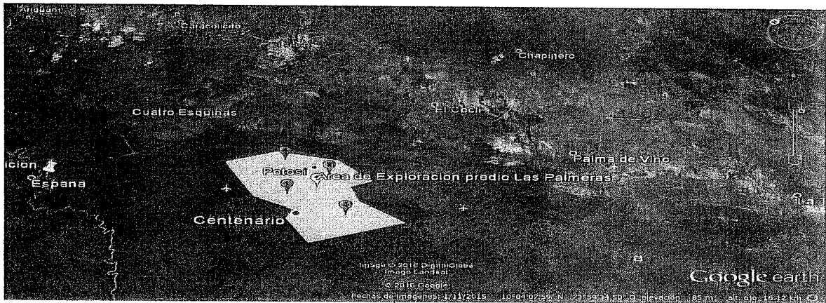
Georreferenciación del Área de Exploración
