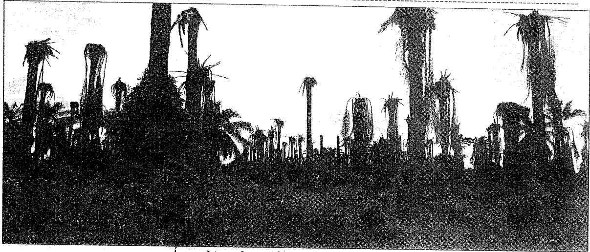
Área de exploración predio Las Palmeras
